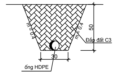
MẶT CẮT CHÔN ỐNG ĐẠI DIỆN Tỷ lệ 1-20
